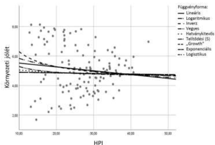
3. ábra: A boldog bolygó mutató és a környezeti jólét mutatójának kapcsolata a teljes mintában
